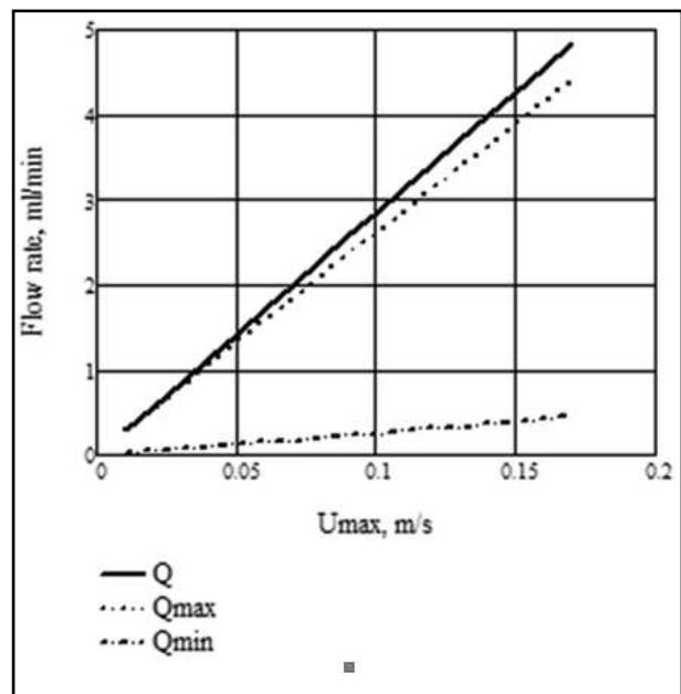
Рис.2. Изменение расхода в различных частях дихотомии 2 типа в зависимости от скорости кровотока
