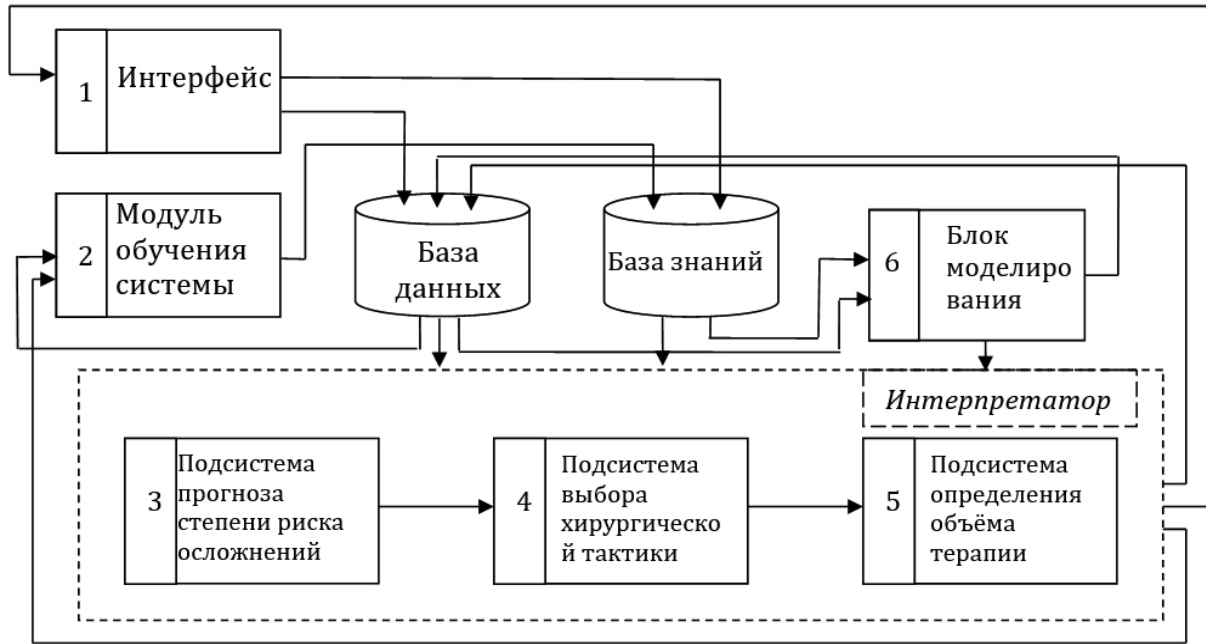
Рисунок. Структурная схема ЭСПОР.
